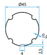
A3505_0504 Adapteri za cijevi ZF 45
