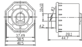
A3515_5179 Osmerokutna remenica 40 u stanju mirovanja
