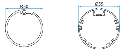
A3505_0517 Adapteri Okrugli Hunter Ø50 užlijebjeni - Okrugao Ø55 Zanzar System
