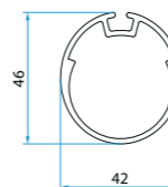
A3505_0508 Adapteri za ovalne cijevi 42x46
