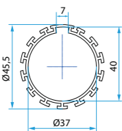
A3505_0510 Adapteri za okrugle cijevi 40 deb. 1,5 mm sa zupcima
