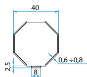
A3505_0501 Adapteri za osmerokutne cijevi 40 (vanjska kopča)
