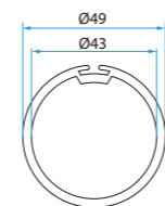
A3505_0513 Okrugli adapteri Mottura Ø 49
