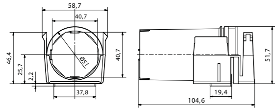
A3516_5180 Uređaj za zavijanje s držačem
